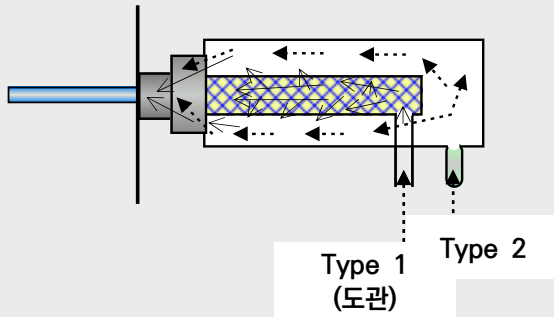
〈그림〉 시료채취부 퍼지방법
